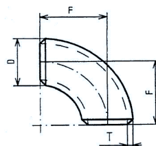
KOLENA 90° 3D (r=1,5xD) EN 10253-4
